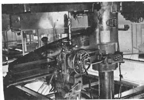
Een boormachine waar men in de werkplaats altijd erg gelukkig mee is geweest en nog is, is deze stoere radiaal-boormachine, die gaten kan boren tot 100 mm. De boor zwenkt om een kolom. Het werkstuk hoeft dus niet verplaatst te worden bij het boren van meerdere gaten. Dit is vooral bij grote en zware werkstukken zeer belangrijk.
