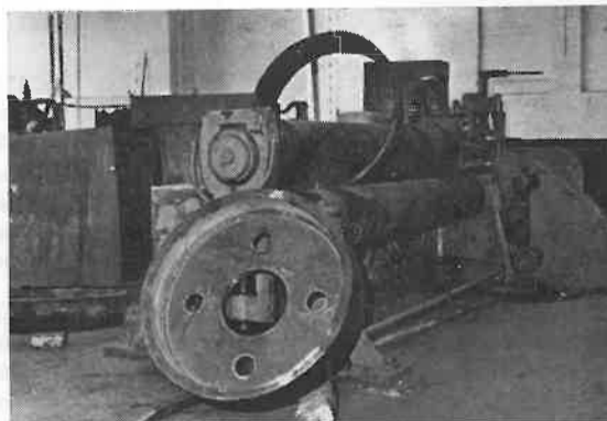
Op deze foto ziet u in 2 onderdelen een tandwiel (vang) in wording. Dit wiel heeft een doorsnede van 1.07 meter. Het onderdeel op de wals wordt hier konisch gewalst. Plaat van 25 mm. dikte kan op deze wals worden bewerkt. De lengte van de wals is 2.50 meter.
