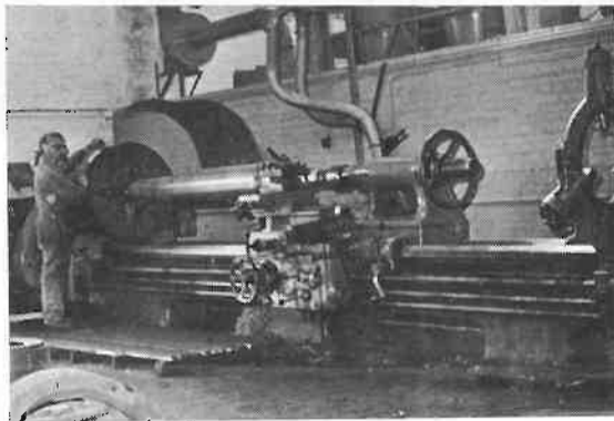
De heer Jac. Huibers aan de grote broer onder de draaibanken. De afstand tussen de centers van deze draaibank kan tot 6 meter worden ingesteld.
