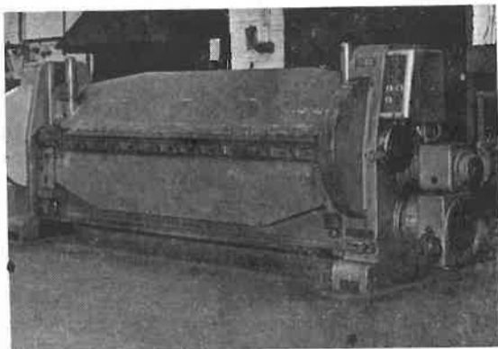
Deze machine is een zetbank. Hiermee buigt (zet) de vakman plaat tot een dikte van 6 mm en een maximale lengte van 2.50 meter in elke gewenste hoek. Na instelling doet deze machine zelfs automatisch zijn werk.
