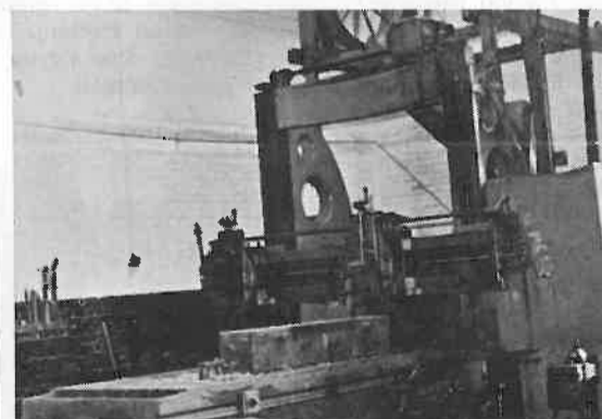
De slee-schaafbank. Met deze schaaftank kunnen oppervlakten bewerkt worden van 2.50 x 1.50 meter en een hoogte tot 70 cm. Een oude getrouwe waar men nog steeds veel plezier van heeft.
